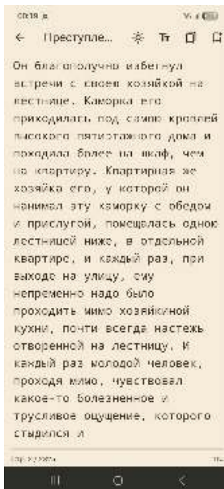
Рисунок 42 – Измененный шрифт
