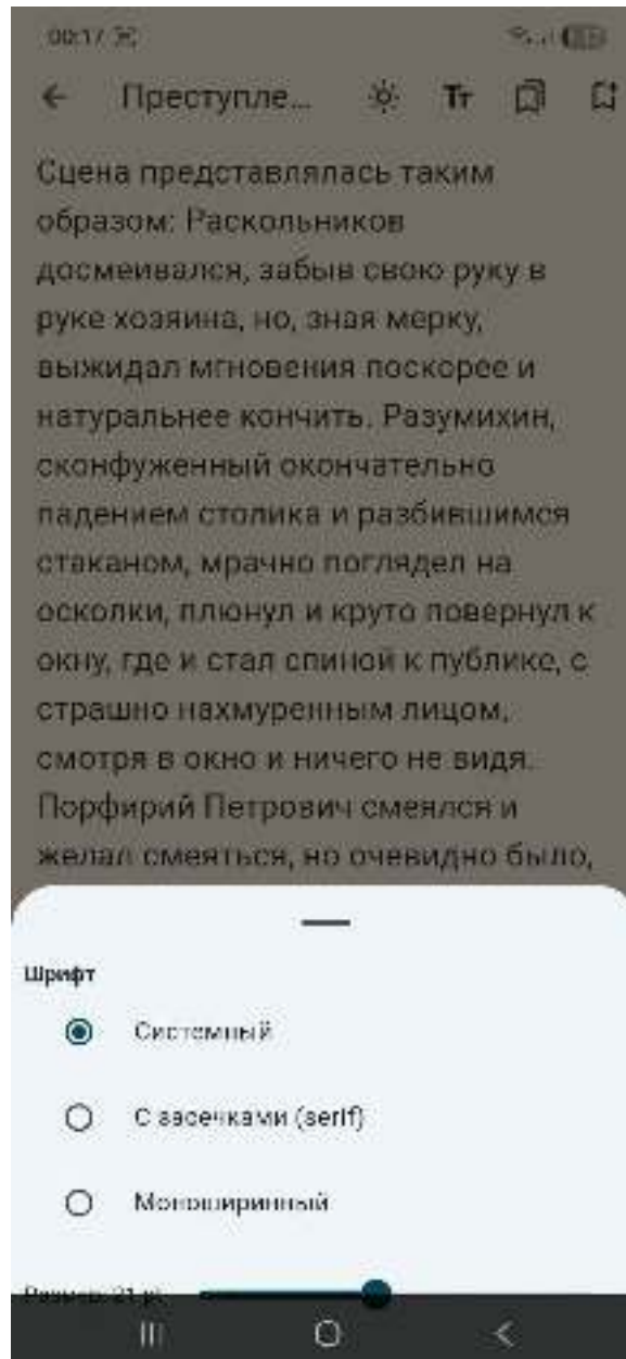
Рисунок 41 – Выбор шрифта
