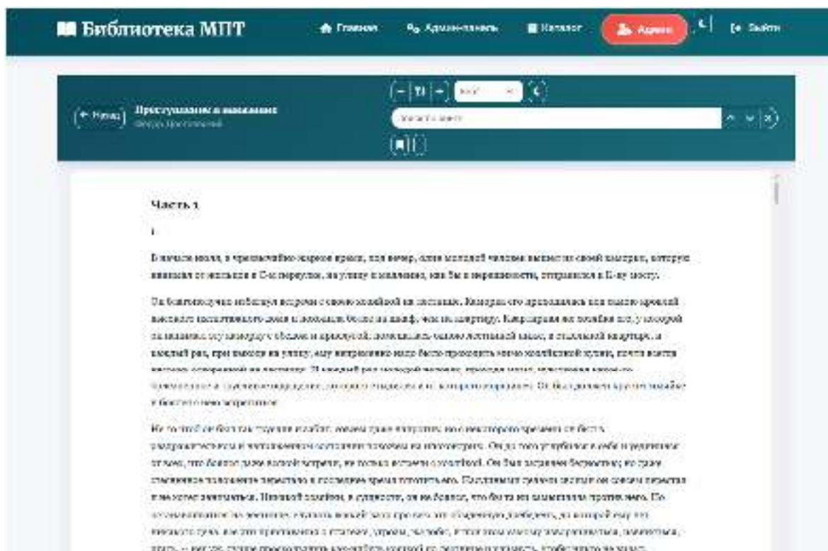
Рисунок 17 – Интерфейс онлайн-читалки
