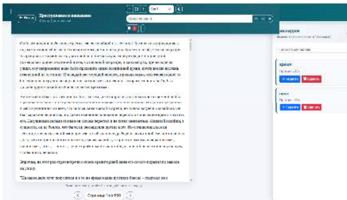
Рисунок 18 – Панель закладок
