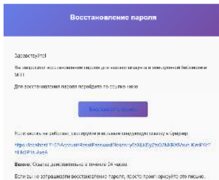
Рисунок 26 – Восстановление пароля
