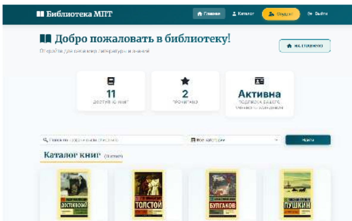
Рисунок 8 – Каталог библиотеки
